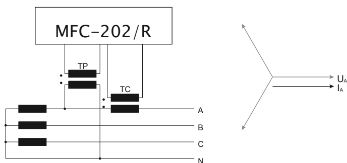
Figura 6.2 Circuito Fase-Neutro, defasagem 0°
