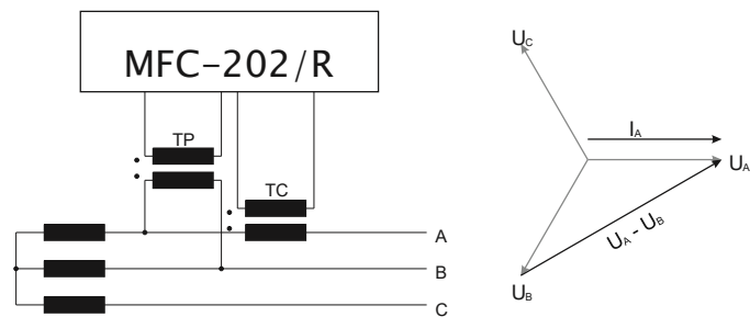
Figura 6.3 Circuito Fase-Fase, defasagem 0^\circ
