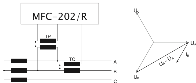
Figura 6.6 Circuito Fase-Fase, defasagem 330^\circ
