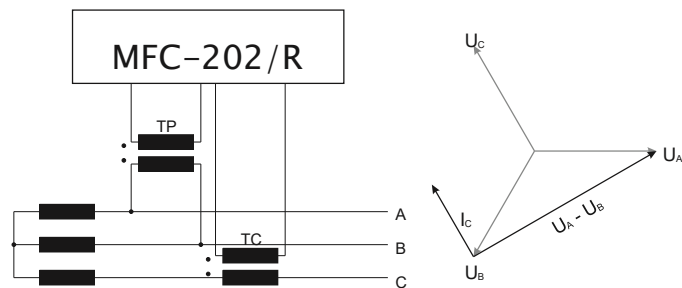
Figura 6.4 Circuito Fase-Fase, defasagem 30^\circ
